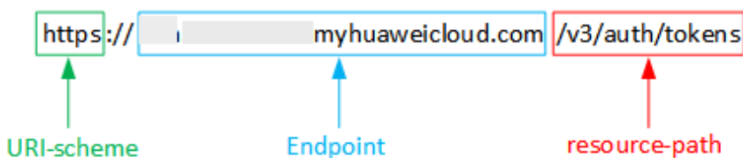
图 3-1 URI 示意图
